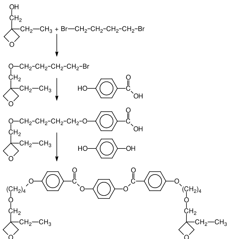
الشكل (16-6): اصطناع مونوميرات أوكسيتان مُحَمَّلة بالوظائف
